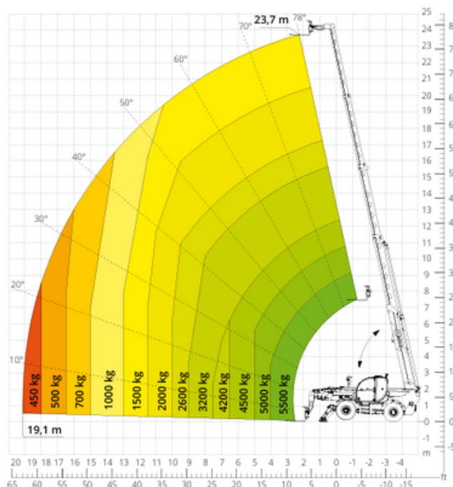
Dodatak viljuška sa korišćenjem stabilizatora
