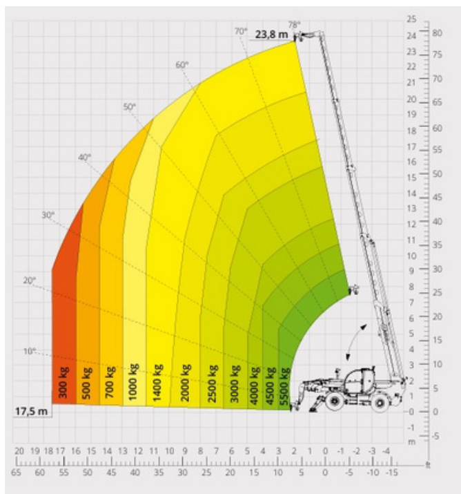
DODATAK KUKA 6.000KG
