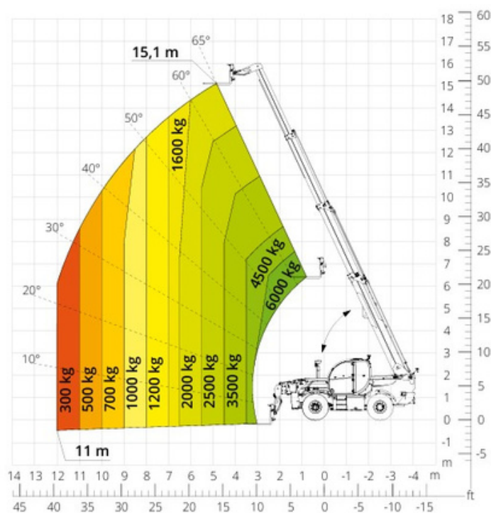
Dodatak viljuška bez korišćenja stabilizatora
