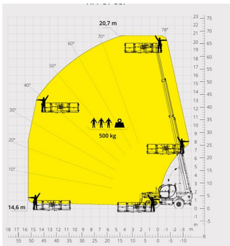
DODATAK ROTIRAJUĆA PRODUŽIVA PLATFORMA 500KG
