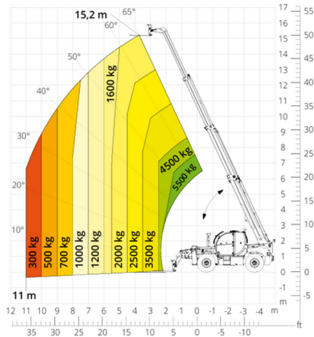
Dodatak viljuška bez korišćenja stabilizatora
