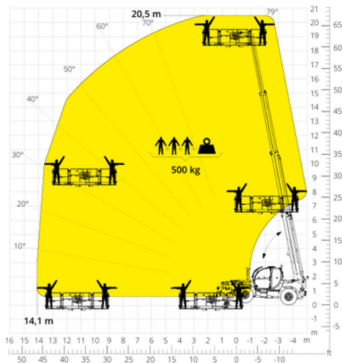
Dodatak proširiva platforma 500kg
